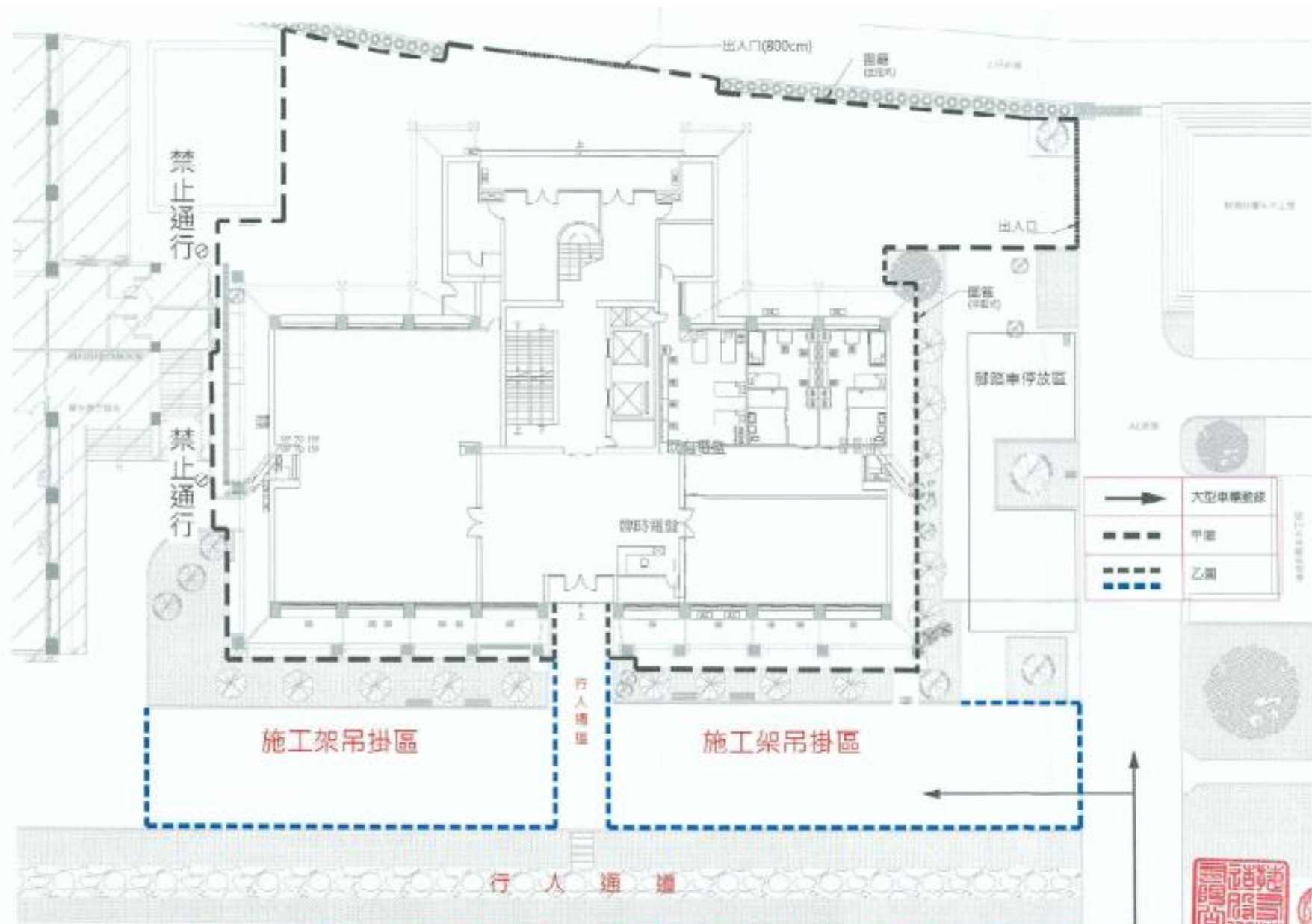
施工架吊掛借用區域封閉平面圖
